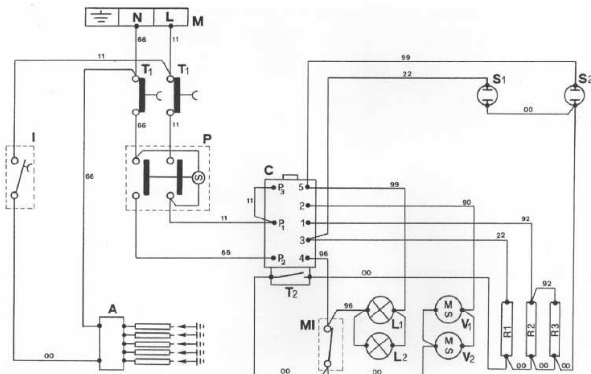
SCHEMAT IDEOWY MODELU KCV 96 P
